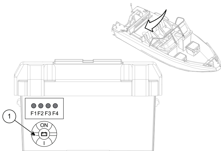
Figur 8.1 Hovedbryter og sikringspanel i Buster X
