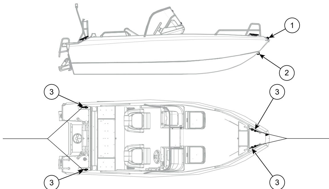
Figur 5.5 Fortøynings- og slepepunkter for Buster X
