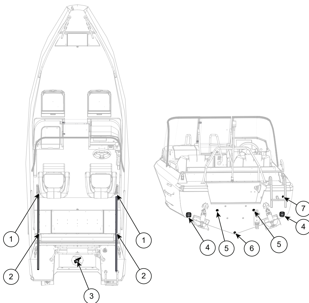
Figur 9.1 Dreneringsutstyr i Buster X
